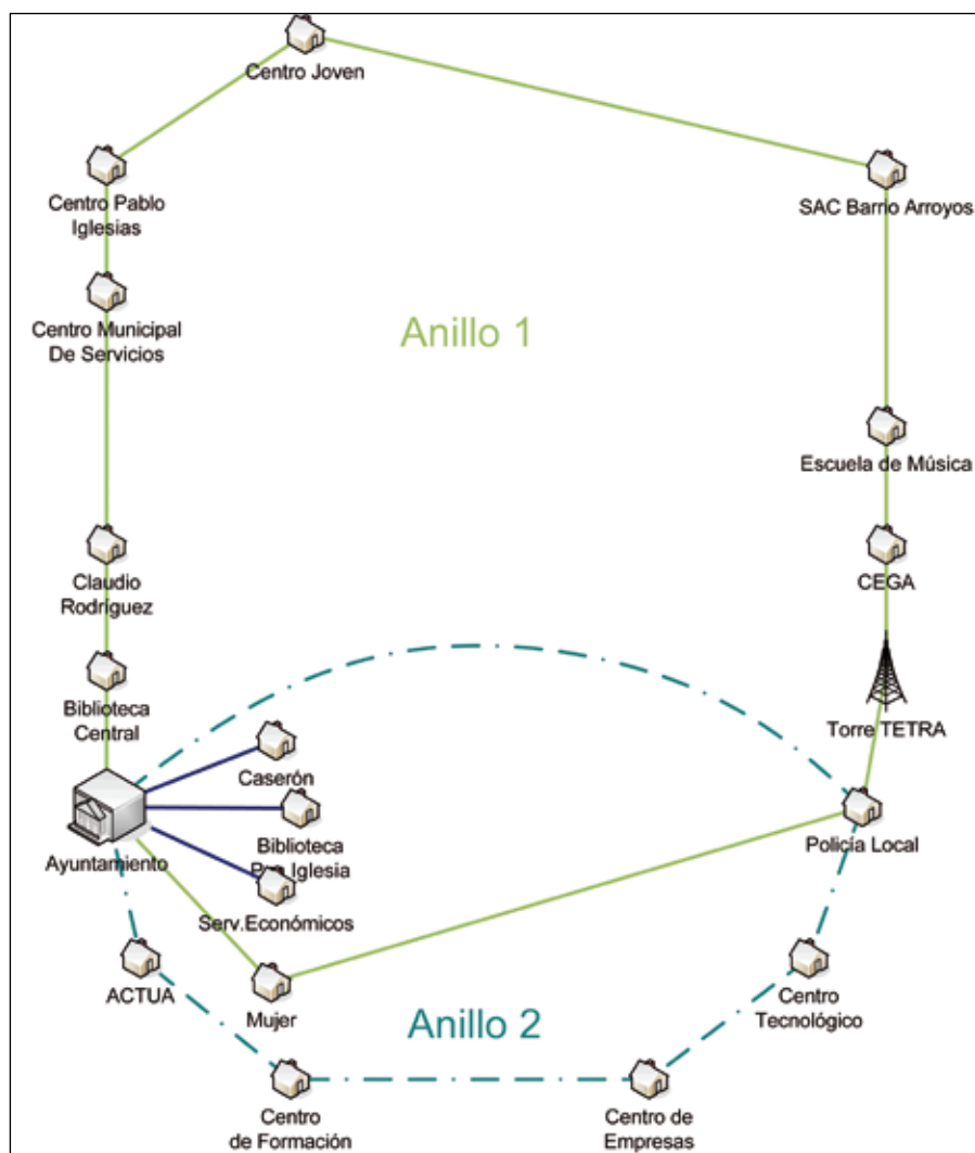
Conexión mediante fibra óptica de "Edificios Principales" (Se incluyen las sedes - Caserón, Biblioteca "Plza. La Iglesia" y Servicios Económicos - conectadas actualmente mediante fibra óptica propia).
